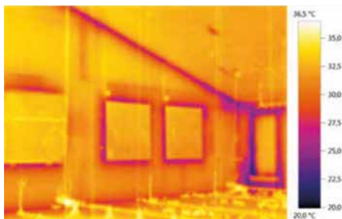
Foto 11: panelen voor de profielen gezet in de kopgevel, geeft duidelijk minder koudebruggen.
