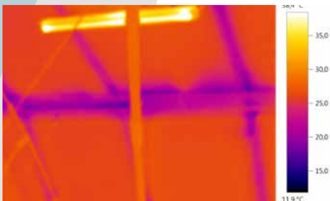
Foto 9: de nok vormt een lange koudebrug in de stal, dit kan leiden tot neerslaande koude lucht op het strooisel.
