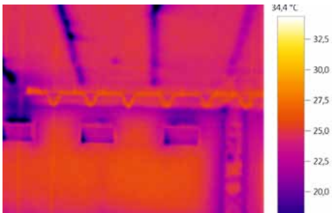
Foto 8: een nieuw plafond met strips is geen garantie voor een plafond zonder koudebruggen!
