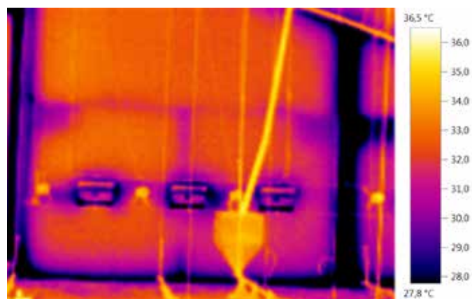
Foto 10: de panelen van de kopgevel zijn tussen de spanten geplaatst met een brede koudebrug tot gevolg.
