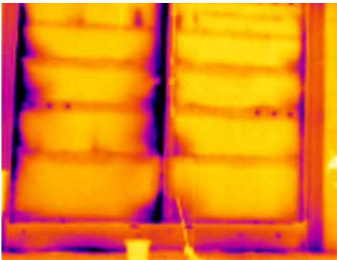
Foto 13: sectionaalpoorten raken verwrongen, waardoor veel warmte verloren gaat.
