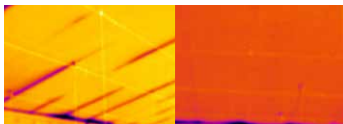
Foto 7: voor: het bijwerken van de kieren tussen de isolatieplaten geeft een mooi resultaat.
