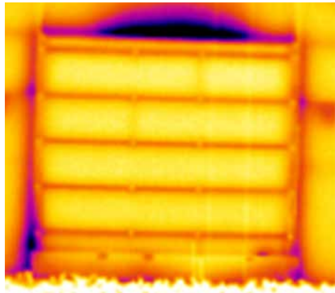
Foto 13: sectionaalpoorten raken verwrongen, waardoor veel warmte verloren gaat.
