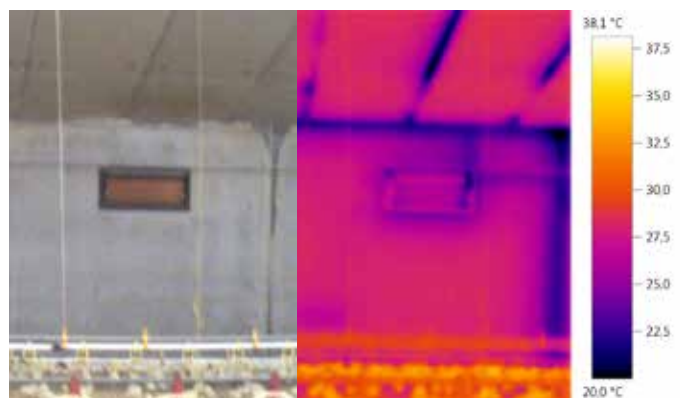
Foto 4: panelen zijn voor spanten geplaatst, toch is er nog een donkere band met koudebrug te zien op het IR-beeld. Rechts van het inlaatventiel zit een fout in de isolatie.
