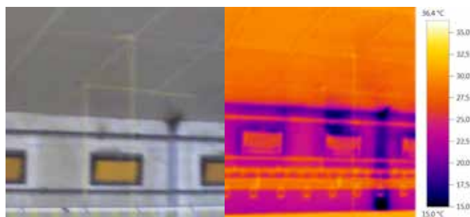
Foto 3: links de digitale foto, rechts het infraroodbeeld. De zichtbare spanten vormen een zware koudebrug met een brede donkerblauwe streep, omdat de betonpanelen tussen de spanten geplaatst zijn.
